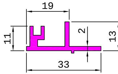
25060 0.336 kg/m
