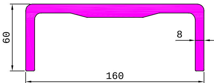
25144 6.401 kg/m
