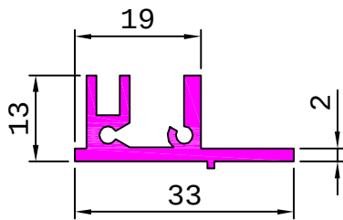
25059 0.371 kg/m
