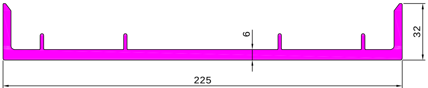
25129 4.438 kg/m
