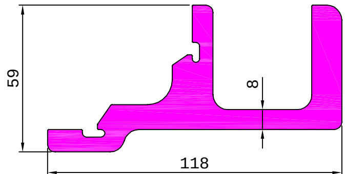
25143 5.654 kg/m
