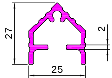
25129 4.438 kg/m
